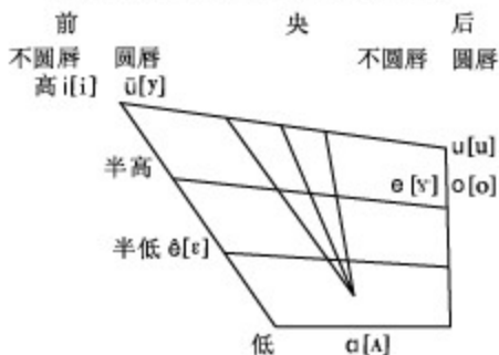
普通话舌面单元音韵母舌位唇形图
